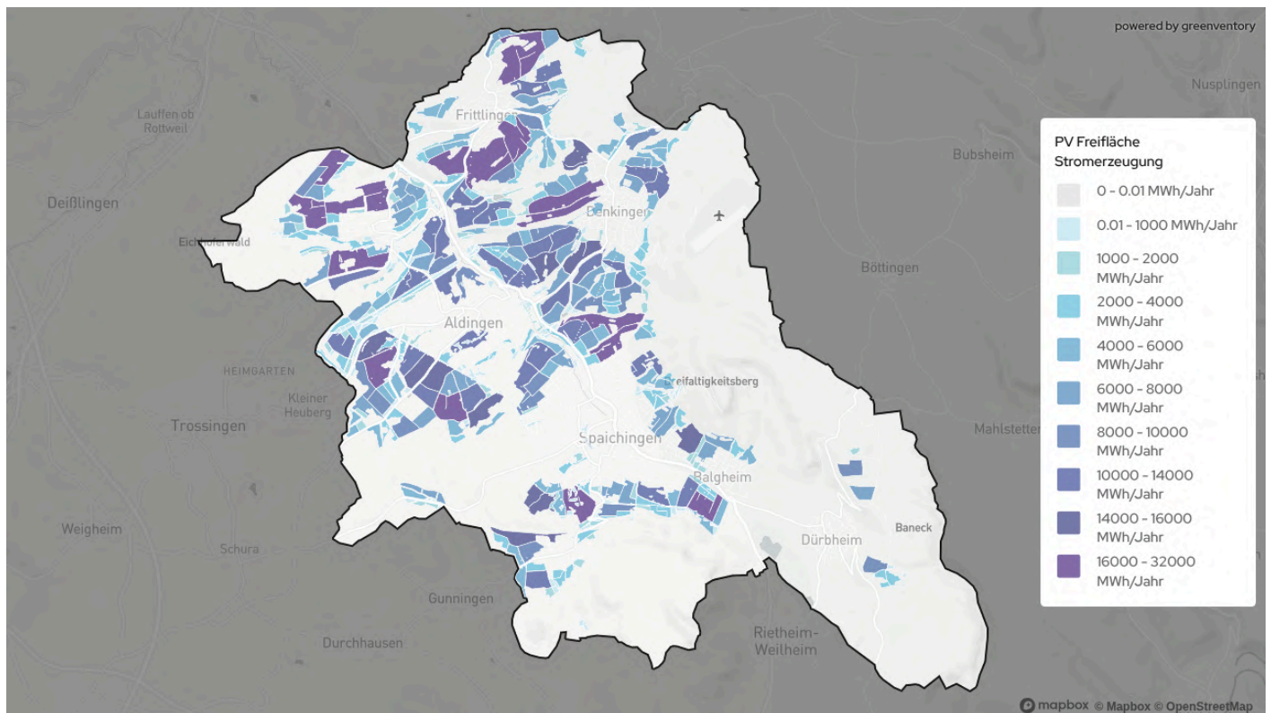
Abbildung 22: Technische Potenzialflächen für Photovoltaik auf Freiflächen
