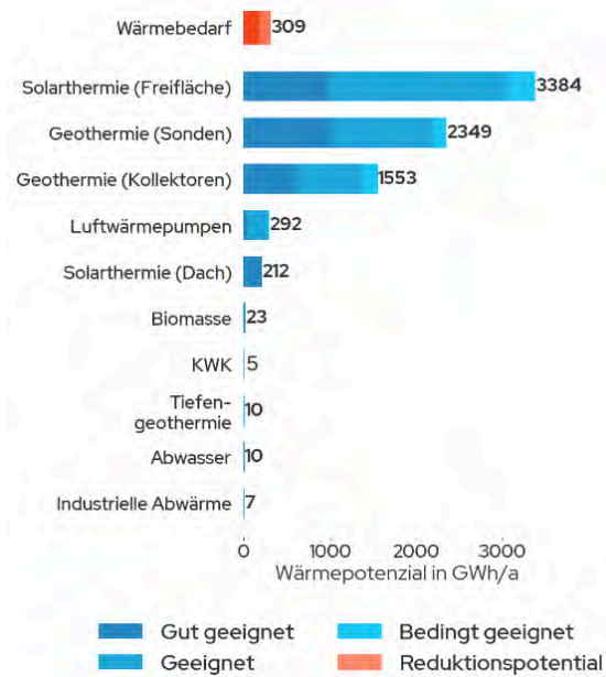
Abbildung 33: Erneuerbare Wärmepotenziale im Projektgebiet
