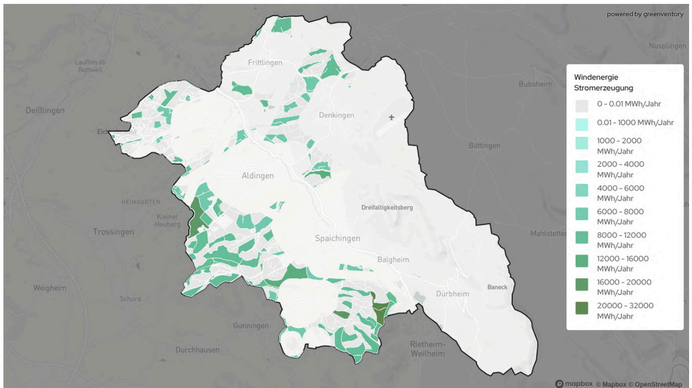
Abbildung 21: Technische Potenzialflächen für Windkraft
