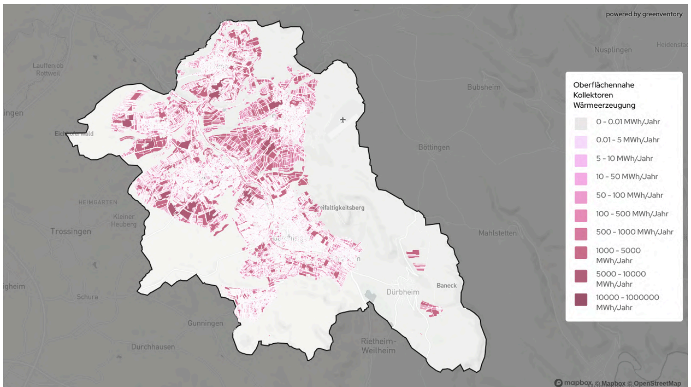
Abbildung 29: Technische Potenzialflächen für Geothermie-Kollektoren
