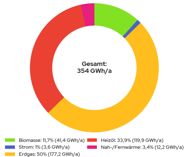
Abbildung 13: Endenergiebedarf nach Energieträger
