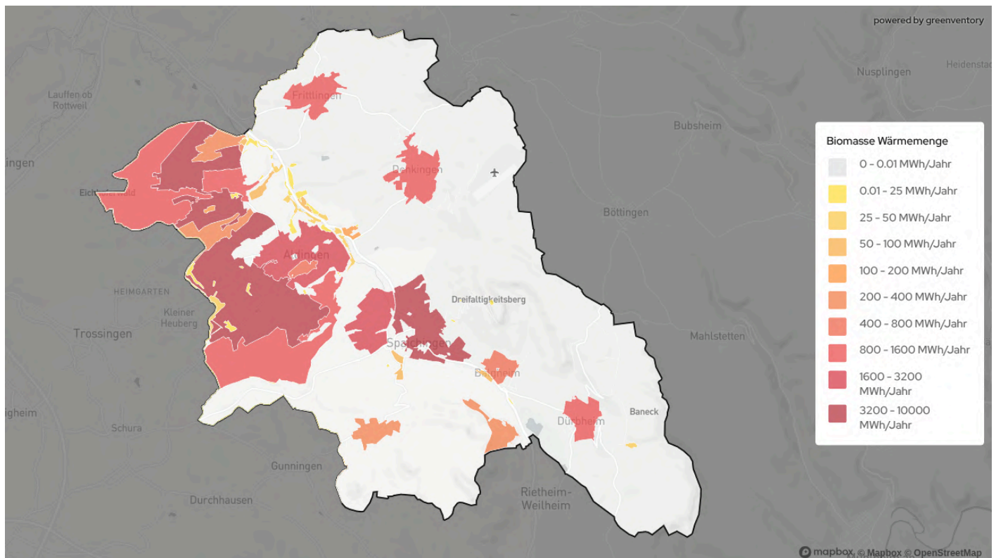
Abbildung 30: Technische Potenzialflächen für Biomasse
