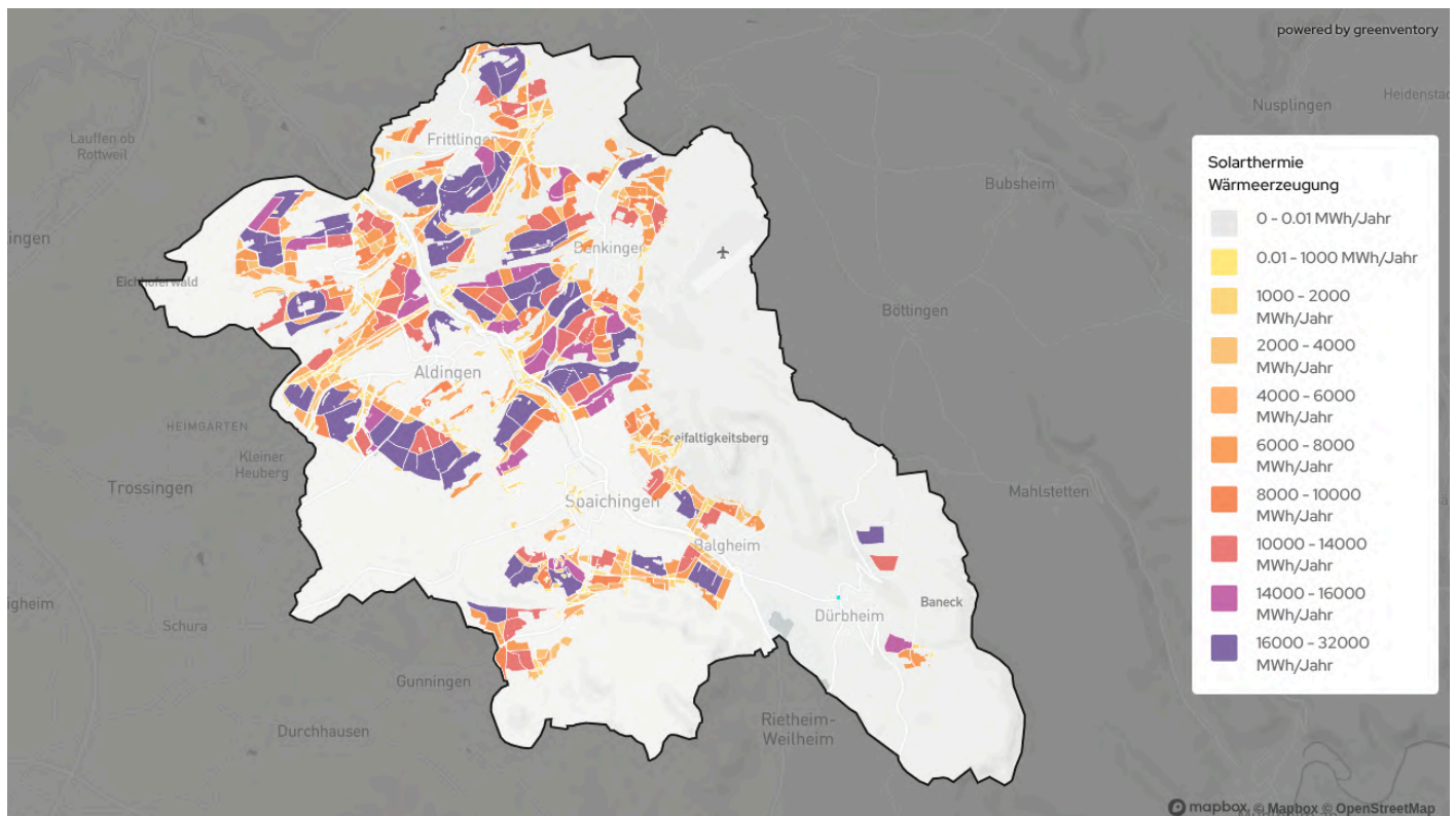
Abbildung 25: Technische Potenzialflächen für Solarthermie auf Freiflächen
