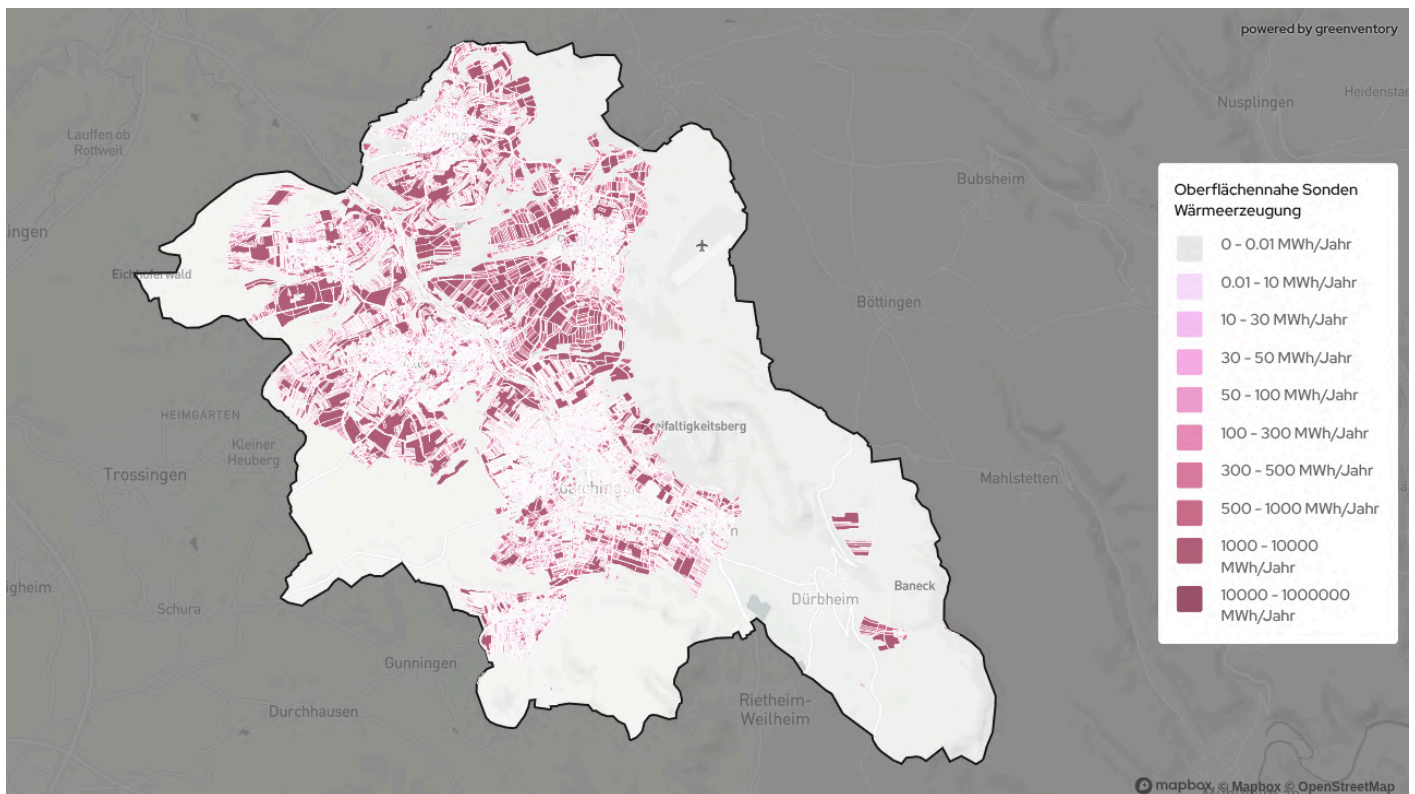
Abbildung 28: Technische Potenzialflächen für Geothermie-Sonden
