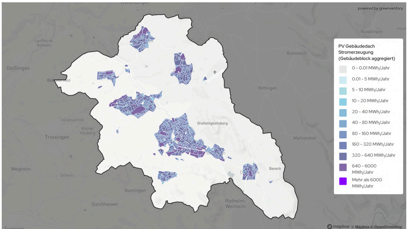
Abbildung 23: Technische Potenzialflächen für Photovoltaik auf Dachflächen
